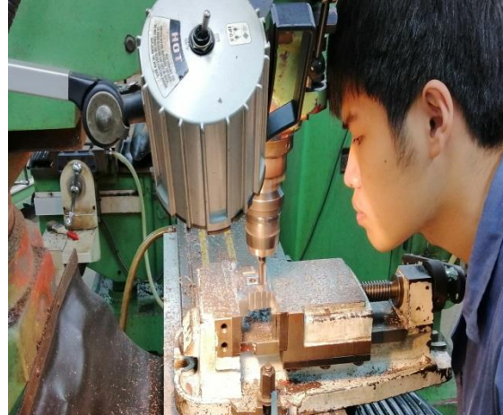
圖(22) 模具固定板製作
