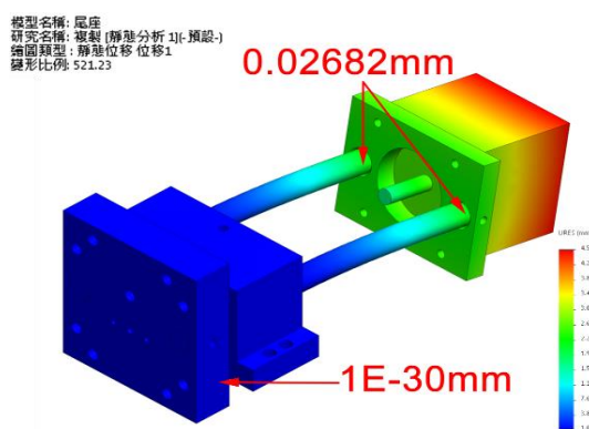
圖(15) 開模變型量
