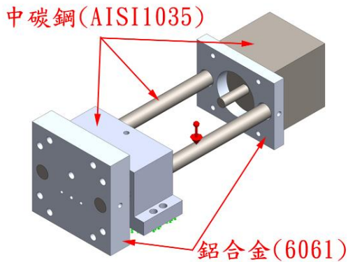
圖(13) 材料設定
