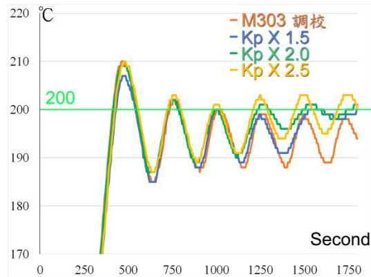
圖(31)M303 K_p 不同比例比較
