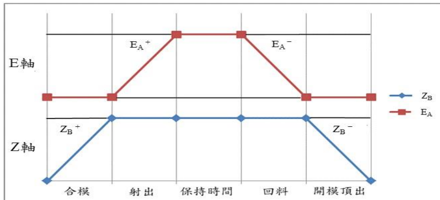
圖(26) 步進馬達的動作時序圖
