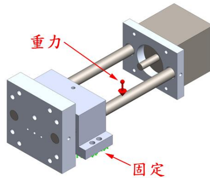
圖(14) 受力條件
