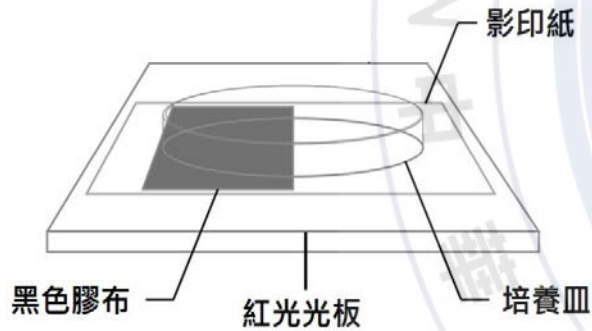
圖3A 紅光偏好測試裝置示意圖
