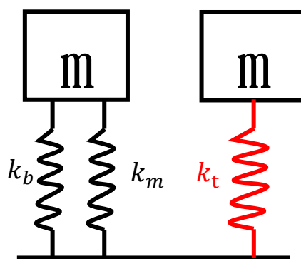
圖 30：並聯彈簧機械模型
