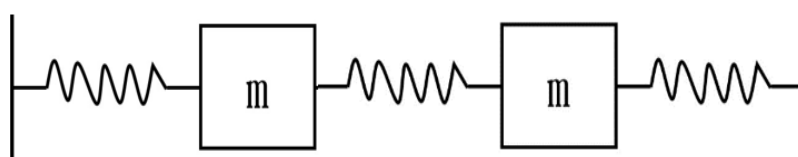
圖 33：兩質量+三彈簧振動模型
