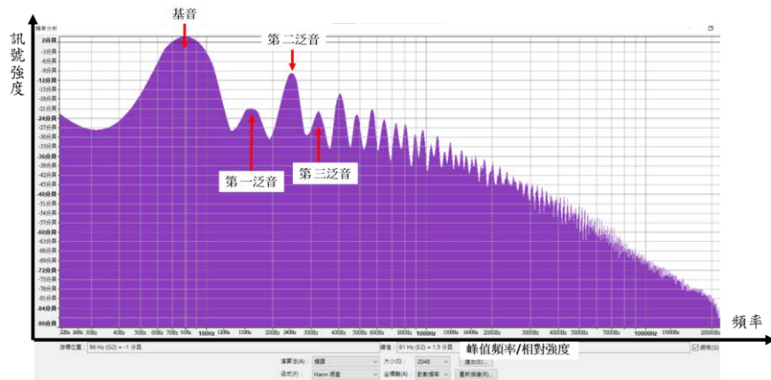
圖15：頻譜分析
