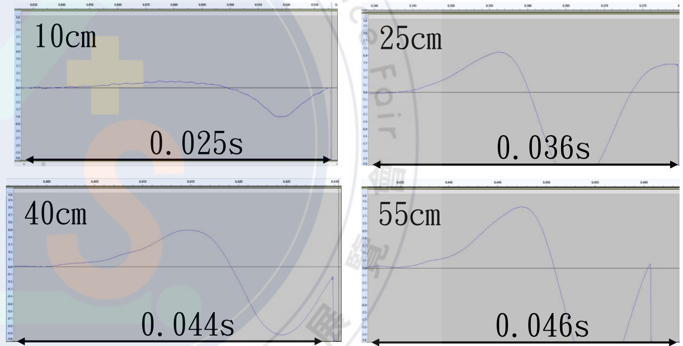
前段波形
