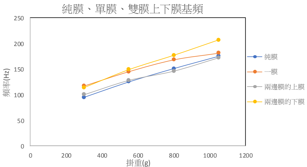
圖 334：純膜、單膜、雙膜上下膜基頻
