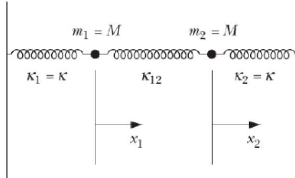
圖 13：耦合振動
