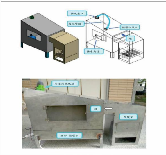
圖 8. 第三代細部設計與完成品
