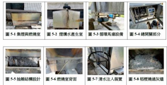
圖5. 第二代煙燻水內部構造
