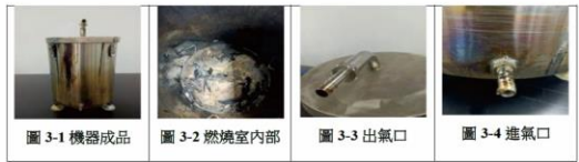
圖3. 第一代煙燻水內部構造
