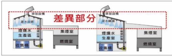
圖 6. 第二代與第三代設計差異部分。
