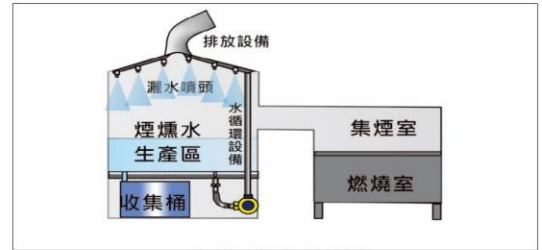
圖4. 第二代煙燻水設計初稿
