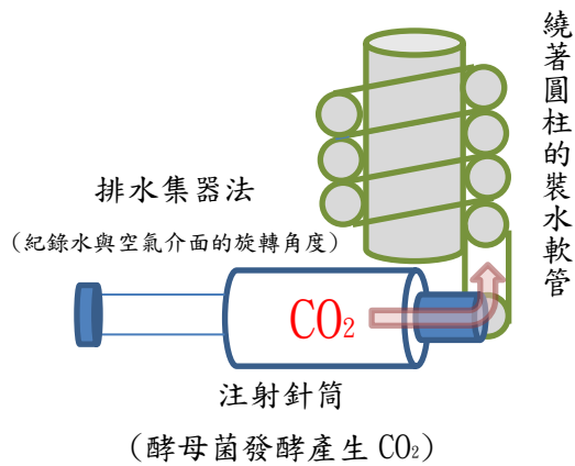
圖五：Y-CO 2 儀器原理說明圖
