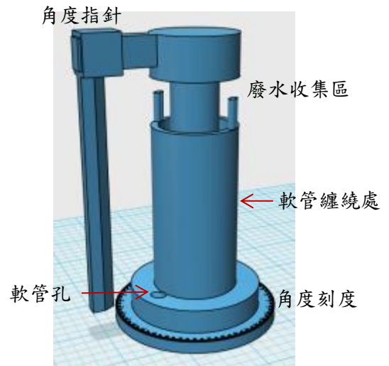
圖六：Y-CO 2 儀器 示意圖
