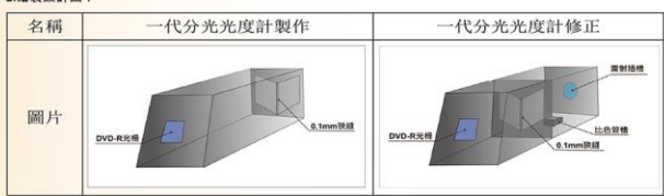
圖23. 第一代分光光度計設計圖
