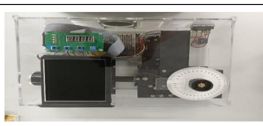
圖 34. 暗箱元件設計
