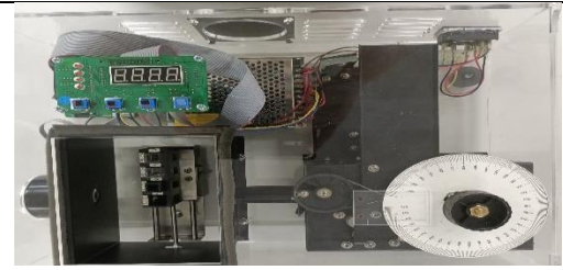
圖 35-2 本研究自製分光光度計
