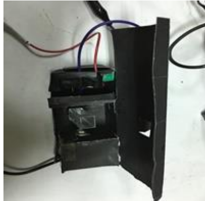
擺放光源盒在比色管另一側，光度儀暗箱蓋可定比色管上方開孔位置
