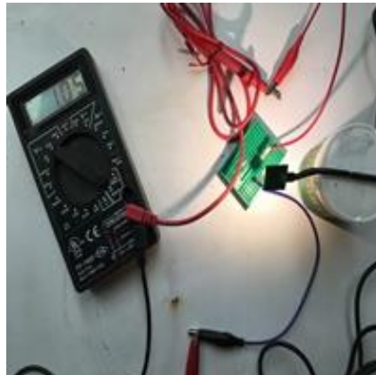
4.5V 電源下光敏電阻照 5V LED 燈的光感應電壓含 180 \Omega 電阻的背景電壓
