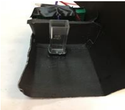
比色管與凹槽放在光敏電阻前的最佳位置上，固定之
