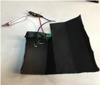
白膠黏結雙層黑紙成光度儀暗箱，先固定光敏電阻和電阻串接的麵包板及觀察測試接線
