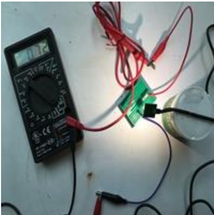
3V 電源下光敏電阻照 5V LED 燈的光感應電壓含 180 \Omega 電阻的背景電壓
